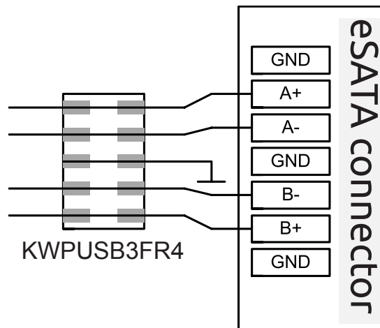
eSATA ESD protection using KWPUSB3FR4
