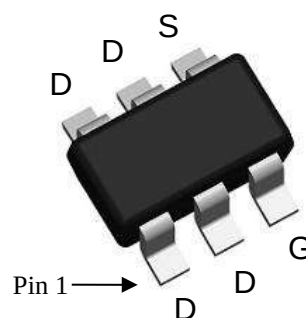
SOT-363
